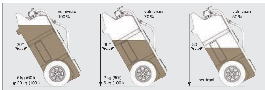
Diesel- en huisbrand olie-Trolley 60 l met snelkoppeling
