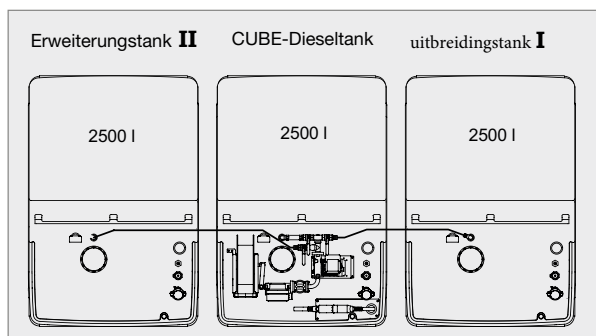
CUBE-dieseltankinstallatie 7.500l met uitbreidingseenheid I en II
