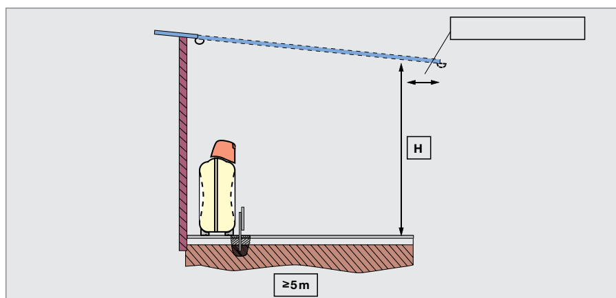
Überdachung für Abfüllplätze
