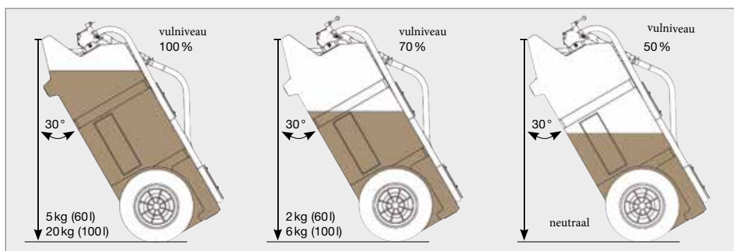
Diesel- en huisbrand olie-Trolley 60l met snelkoppeling, zonder pomp
