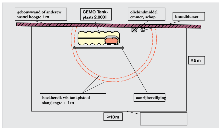
Voorbeeld: eigen verbruik aftankplaats tot 2000 l, zonder dak, zonder afscheider
