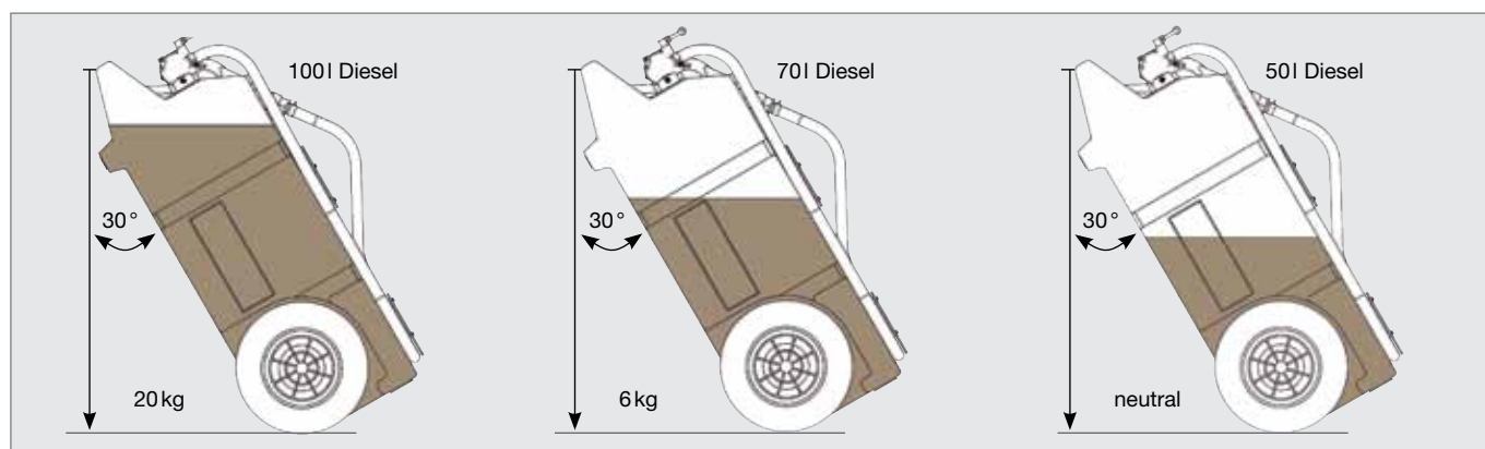
gewichtsbelasting a/d handgreep in de transportstand
