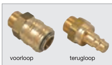
snelkoppelingssset echter met tegenstuk en aansluiting 3/8" buit.schr.draad voor voor- en terugloop passend voor mobiele olietanks en generatoren
