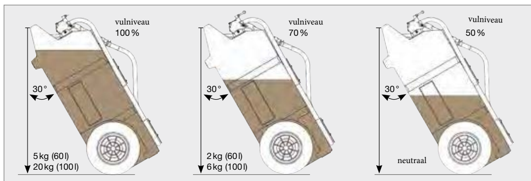
Diesel- en huisbrand olie-Trolley 60l met snelkoppeling, zonder pomp
