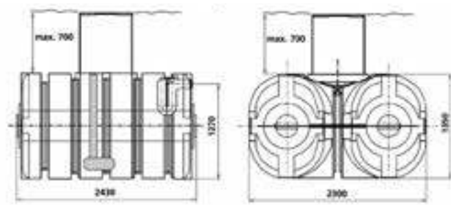
oppervlaktereservoir 5.000l
