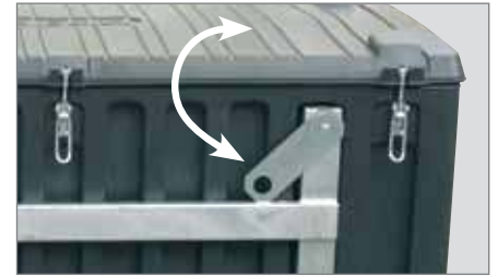
Krangestell mit schwenkbaren Kranösen (bei CEMbox 750 I kranbar)
