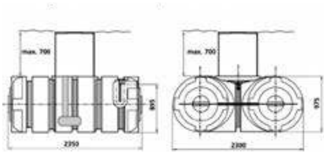
Oppervlaktereservoir 3.500l
