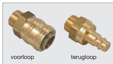
snelkoppelsset echter met tegenstuk en aansluiting 3/8" buit.schr.draad voor voor- en terugloop passend voor mobiele olietanks en generatoren
