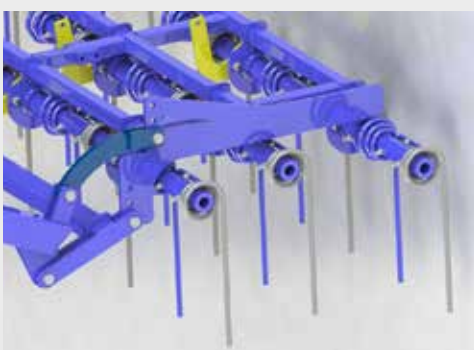
3-rijen stro-eg
