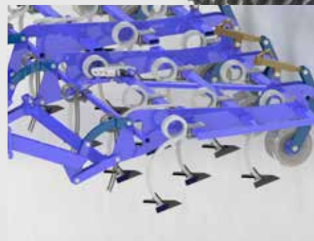
3-rijige Flügelschare
