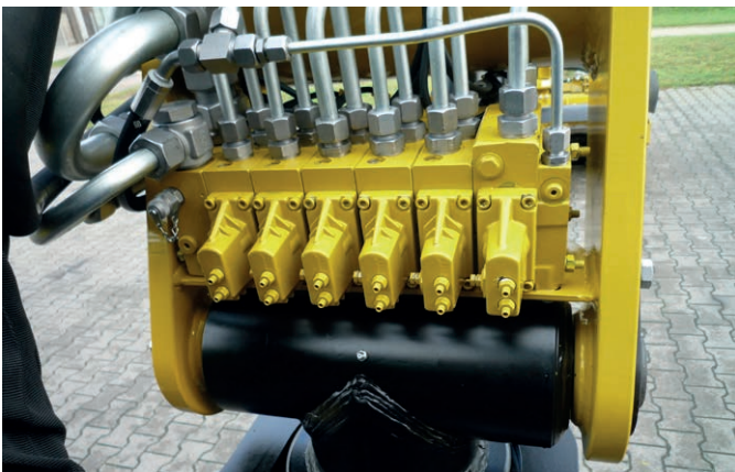
Danfoss Ventilblock montiert auf dem Ausleger > Keine Schlauchverbindung
