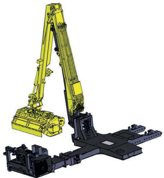
Ausleger mit überfahrbares Rahmen
