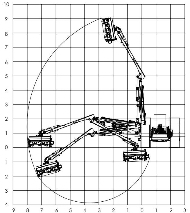
Reichweitentabelle TITAN 7500 mit WMK 1500 Angaben in Meter
