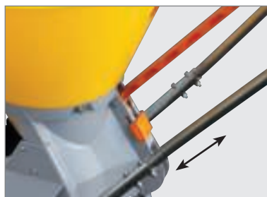
duwstang van RVS, drielukkig in lengte verstelbaar
