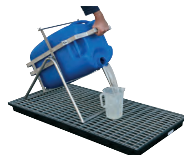
Kanister-Abfüllbock für Kanister bis 60 l
