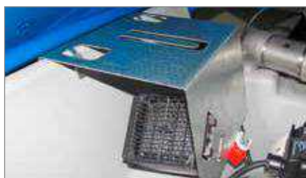
CUBE-tank voor AdBlue®, verwarming en thermostaat
