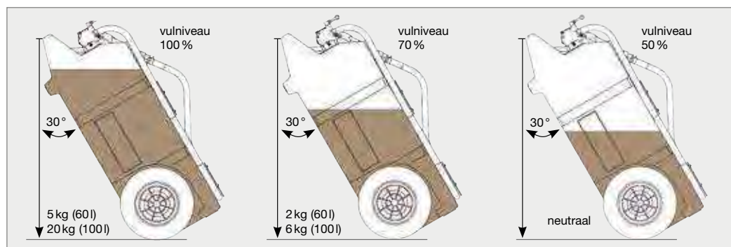
dieseltrolley 100l met handpomp
