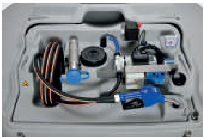
CUBE-tank voor AdBlue®, outdoor Basic
