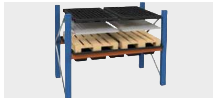
PE plank hangkuip 18/230 voor vakafmetingen 180 x 110 cm
